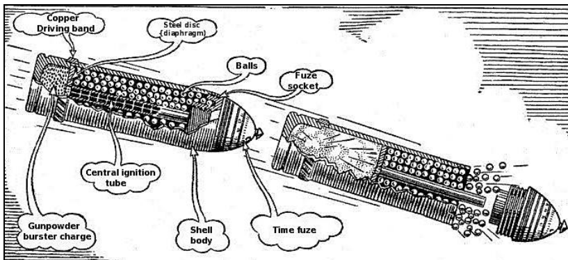
Werking van een schrapnelgranaat. (Uit: Les obus 'Shrapnel', p. 3)
